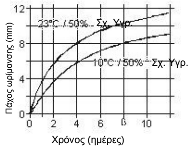
Διάγραμμα 1: Ταχύτητα ωρίμανσης του Sikaflex®-291
